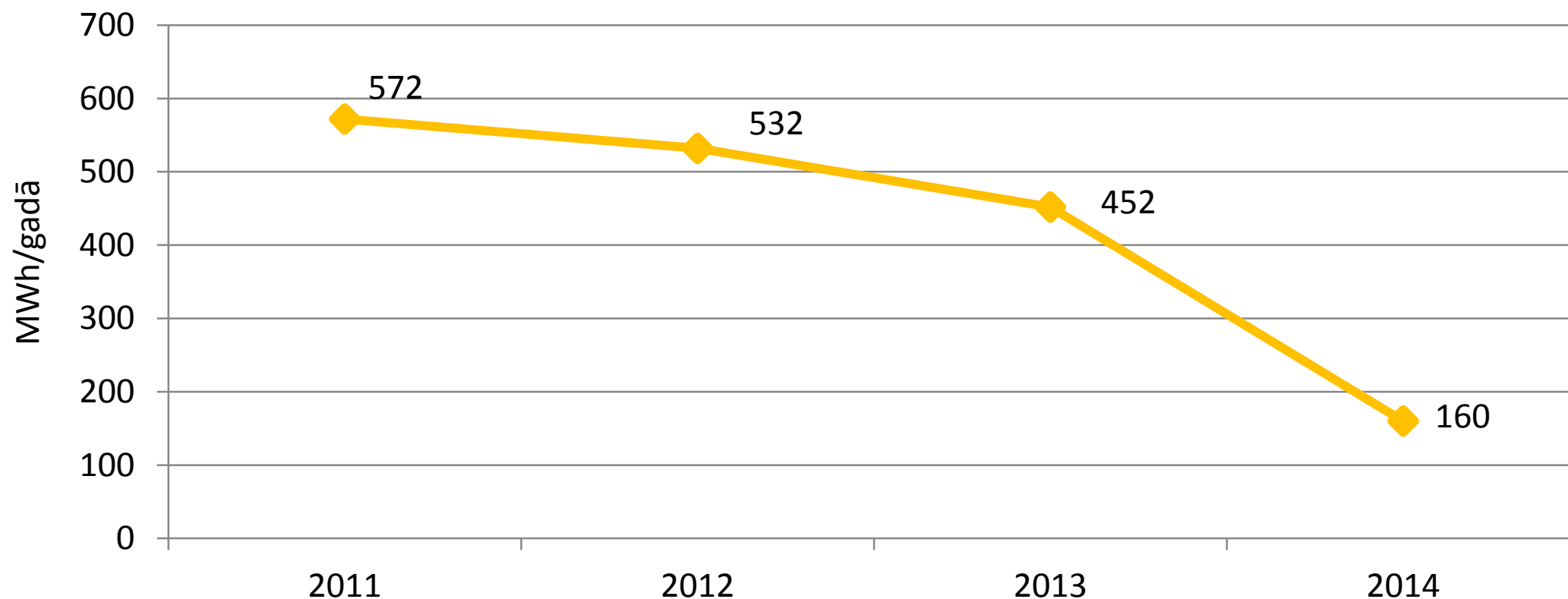
Siltumenerģijas pašpatēriņš 2011.g. – 2014.g.
